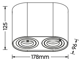
Deckenleuchte · Ceiling lamp excl. 2 x GU10 max. 35 W 612900231 612900232
