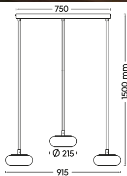
Pendelleuchte · Pendant incl. SMD-LED 3 x 12 W / 3 x 1667 Lumen 4.000 Kelvin 337810331
