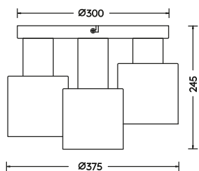
Deckenleuchte · Ceiling lamp excl. 3 x E27 max. 10 W 619430317
