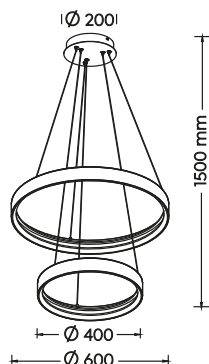
Pendelleuchte · Pendant incl. SMD-LED 37 W / 4.300 Lumen 3.000 Kelvin 355039130
