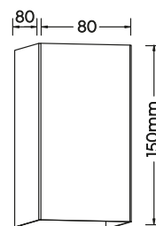
Wandleuchte · Wall lamp excl. 2 x GU10 max. 35 W 206500279
