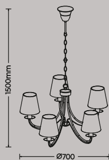
Pendelleuchte · Pendant excl. 5 x E14 max. 28 W 110600531
