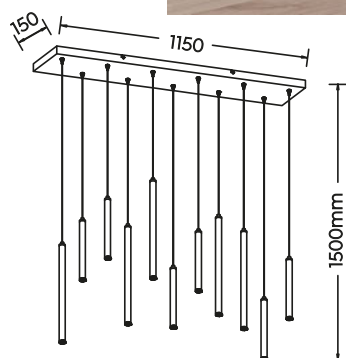
Pendelleuchte · Pendant incl. 11 x SMD-LED 11 x 2,8 W / 11 x 350 Lumen 3.000 Kelvin 321611132
