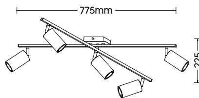
Deckenleuchte · Ceiling lamp excl. 5 x GU10 max. 35 W 612400504 612400580
