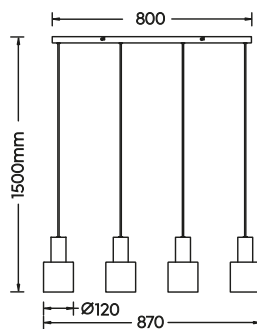
Pendelleuchte · Pendant excl. 4 x E27 max. 10 W 319400417
