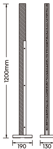
Stehleuchte · Floor lamp incl. SMD-LED 16 W / 1.950 Lumen 3.000 Kelvin 441610132
