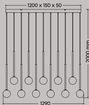
Pendelleuchte · Pendant excl. 11 x G9 max. 5 W 363501117 363501179
