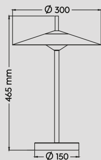
Tischleuchte · Table lamp incl. SMD-LED 12,5 W / 1.400 Lumen 2.300 + 3.000 + 4.000 Kelvin 590810131
