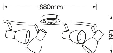
Strahler · Spot incl. 4 x LED E14 4 x 4,9 W / 4 x 470 Lumen 3.000 Kelvin 871010407 871010408
