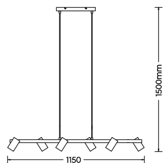
Pendelleuchte · Pendant excl. 6 x GU10 max. 35 W 312490632
