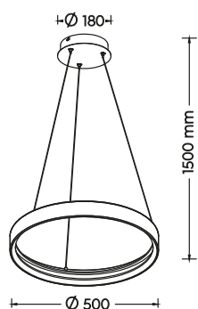
Pendelleuchte · Pendant incl. SMD-LED 28 W / 3.300 Lumen 3.000 Kelvin 355030130
