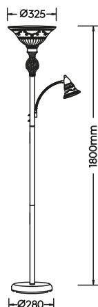
Stehleuchte · Floor lamp excl. 1 x E27, max. 100 W excl. 1 x E14, max. 40 W 4602021-24
