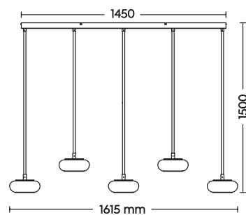
Pendelleuchte · Pendant incl. SMD-LED 5 x 10 W / 5 x 1400 Lumen 4.000 Kelvin 337810531
