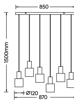
Pendelleuchte · Pendant excl. 6 x E27 max. 10 W 319400617
