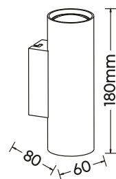
Wandleuchte · Wall lamp excl. 2 x GU10 max. 35 W 212400204
