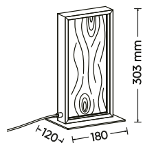
Tischleuchte · Table lamp incl. SMD-LED 10,5 W / 1.150 Lumen 3.000 Kelvin 555510130
