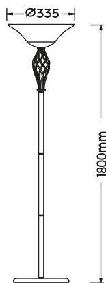
Stehleuchte · Floor lamp excl. 2 x E27 max. 60 W 401000224
