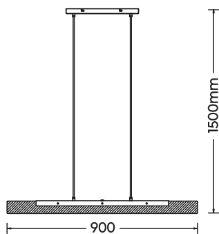
Pendelleuchte · Pendant incl. SMD-LED 25 W / 3.000 Lumen 3.000 Kelvin 341610132
