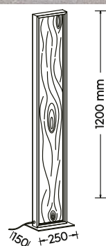
Stehleuchte · Floor lamp incl. SMD-LED 35 W / 4.100 Lumen 3.000 Kelvin 455510130
