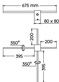
Wandleuchte · Wall lamp incl. SMD-LED 14 W / 1.700 Lumen 2.300 + 3.000 + 4.000 Kelvin 237770131 237770132
