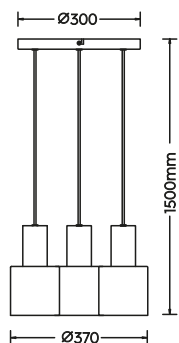
Pendelleuchte · Pendant excl. 3 x E27 max. 10 W 319430317
