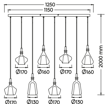
Pendelleuchte · Pendant excl. 8 x E14 max. 10 W 349400817
