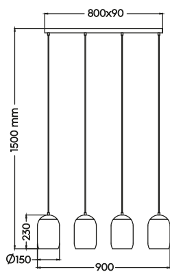
Pendelleuchte · Pendant excl. 4 x E27 max. 10 W 364600417
