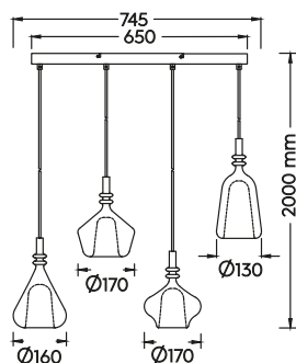
Pendelleuchte · Pendant excl. 4 x E14 max. 10 W 349400417
