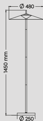
Stehleuchte · Floor lamp incl. SMD-LED 18 W / 2.100 Lumen 2.300 + 3.000 + 4.000 Kelvin 490810131
